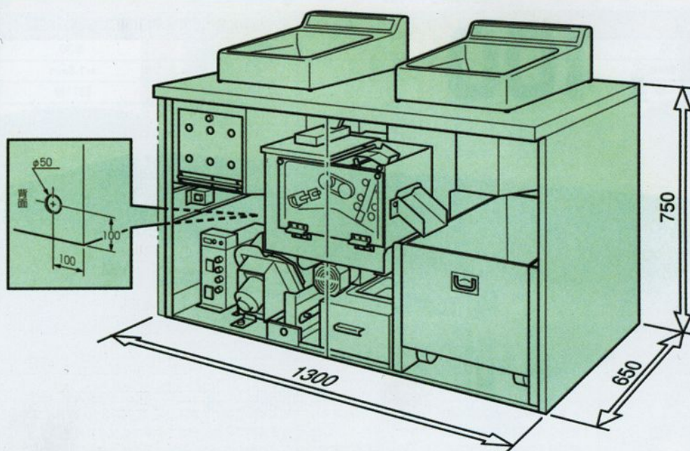
●JT100仕様図
