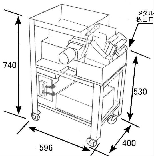
寸法図
